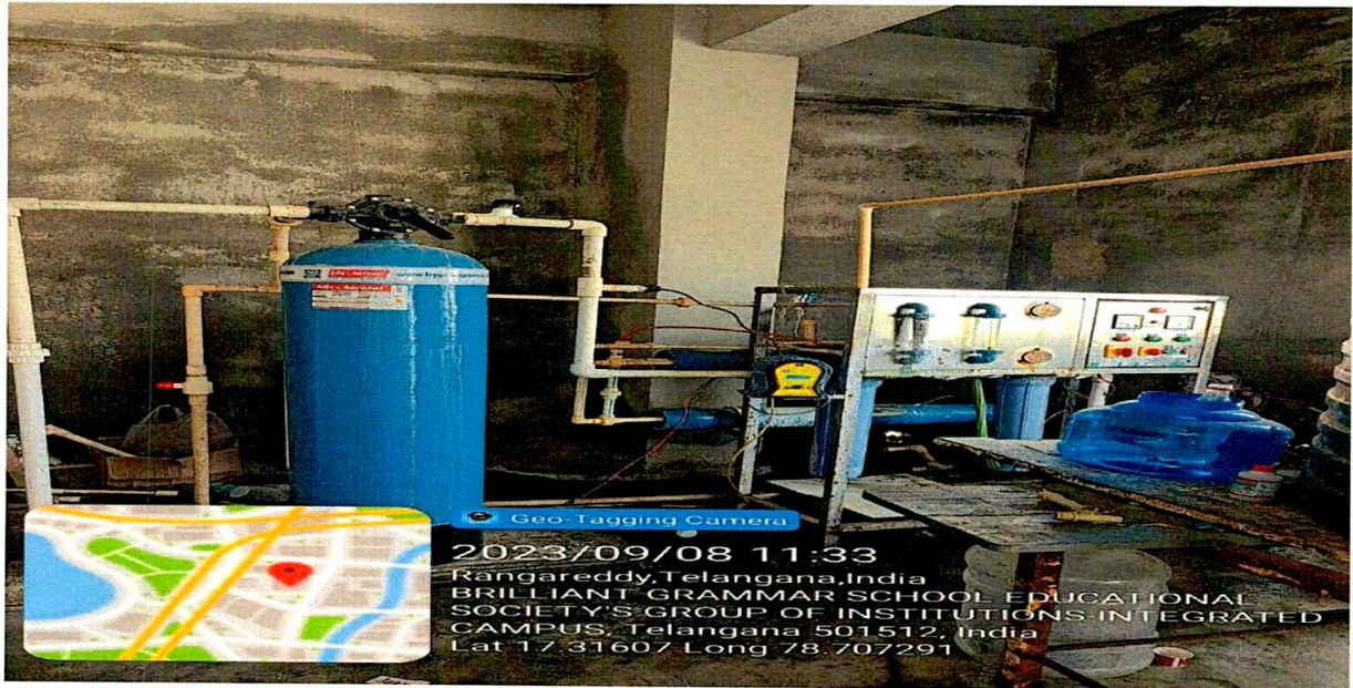
RO Plant.
